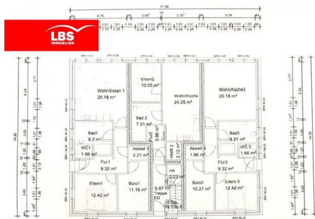
Grundriss Erdgeschoss
