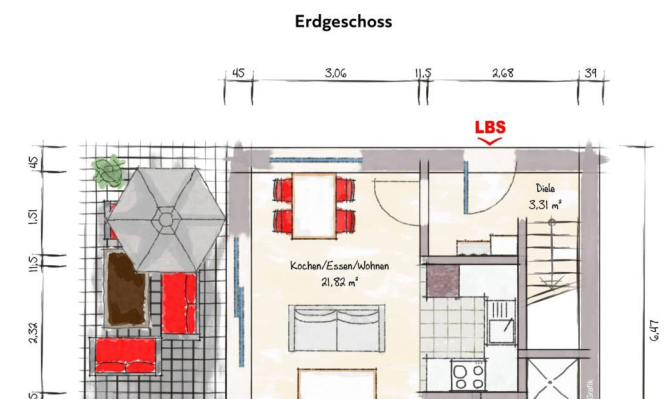
EG Wohnung 10
