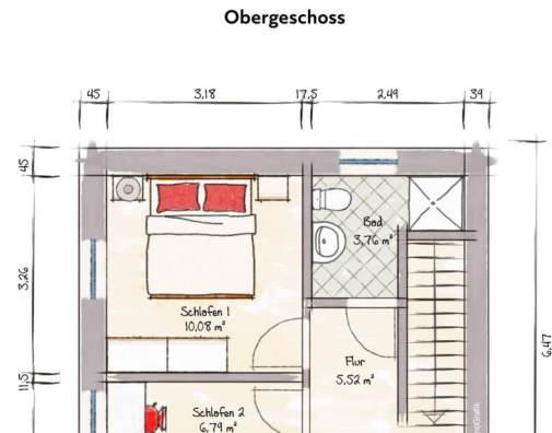
OG Wohnung 10
